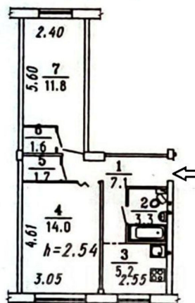
технический план 2-комн. квартиры 44,7 м2
