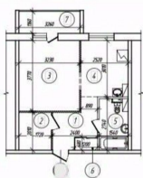
Экспликация помещений после перепланировки
