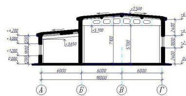
Рис.2. Поперечный разрез здания.
