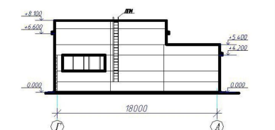
Рис.5. Торцевой фасад здания (в осях Г-А).
