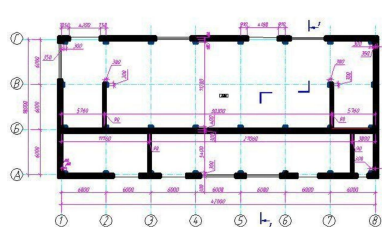
Рис.1. Схематичный план здания.
